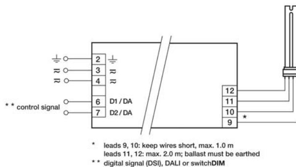
PCA TCL EXCEL one4all 36-80 W
